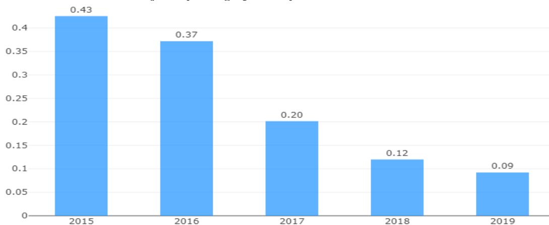
Rysunek 13 Wskaźnik rozwoju – wymiar gospodarczy w Mieście i Gminie Oleśnica w latach 2015–2019
