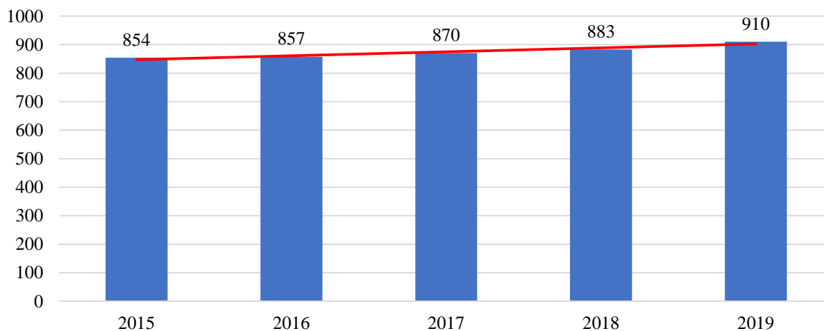
Wykres 10 Podmioty wpisane do rejestru REGON na 10 tys. ludności na terenie MOF Staszowa w latach 2015–2019
