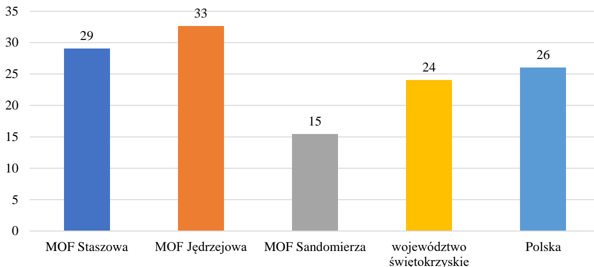
Wykres 9 Pozwolenia wydane na budowę i zgłoszenia budowy z projektem budowlanym w przeliczeniu na 10 tys. mieszkańców dla MOF Staszowa w porównaniu do MOF Jędrzejowa, MOF Sandomierza, województwa świętokrzyskiego oraz Polski w 2019 roku
